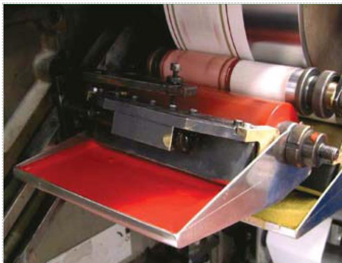
Nettoyage des encres sur les cylindres de flexographie
